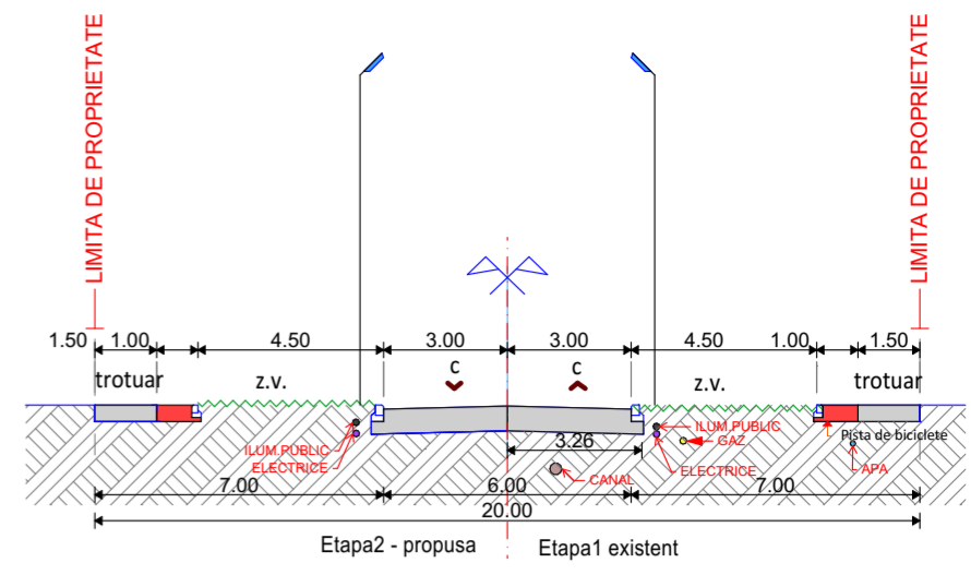
PROPUNERE PROFIL TRANSVERSAL TIP PTT1
