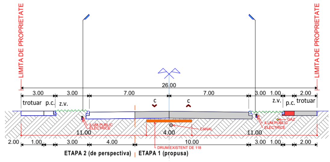
PROPUNERE PROFIL TRANSVERSAL TIP PTT3
