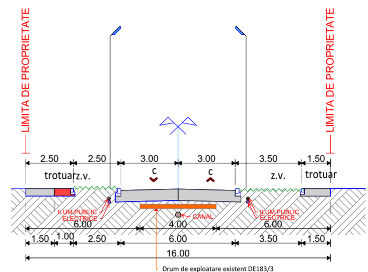
PROPUNERE PROFIL TRANSVERSAL TIP PTT2
